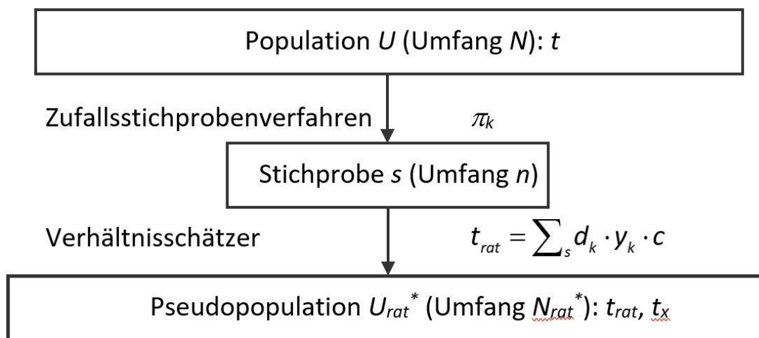
Abb. 4.1 Veranschaulichung der Idee des Verhältnisschätzers als Erzeugung einer Pseudopopulation
